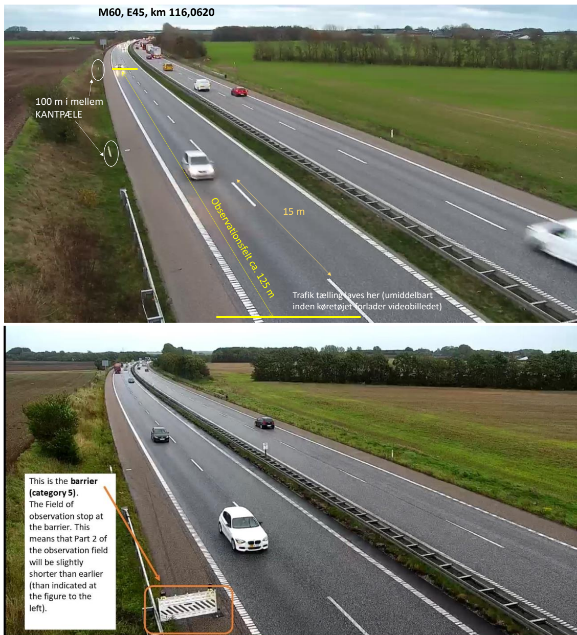
Figur 3. Venstre-drejende kurve M60 - E45, km 116,0620. Horisontal kurveradius er ca. 4.000 m. Øverst: Uden spærrebom i nødspar. Nederst: Med spærrebom i nødspar. Observationsfeltets "startpunkt" bagest i billedet er det samme i begge perioder, mens observationsfeltets "slutpunkt" ender ud for spærrebommen i perioden med spærrebom i nødspar.
