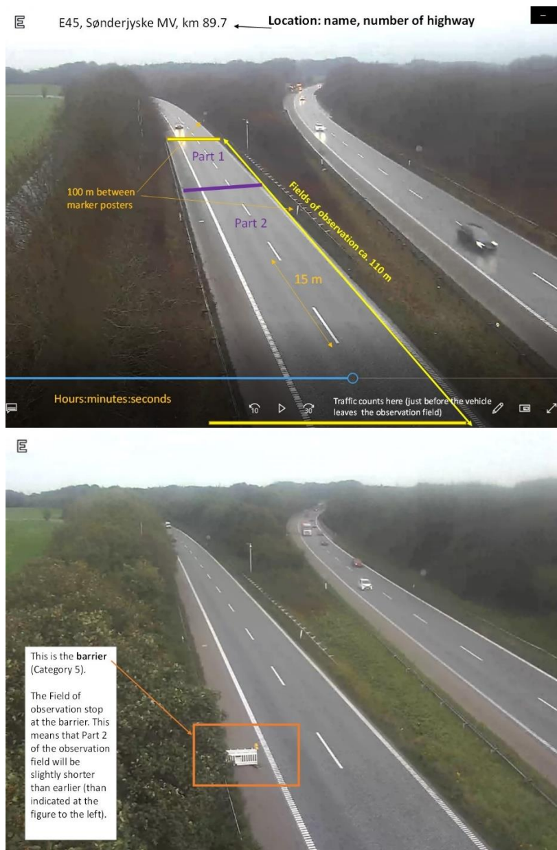
Figur 4. Højre-drejende kurve E45/M50 Sønderjyske MV, km 89,0700, MVX Kolding N, sydgående. Hori-sontal kurveradius er ca. 2.600 m. Observationsfeltets "startpunkt" bagest i billedet er det samme i begge perioder, mens observationsfeltets "slutpunkt" ender ud for spærrebommen i perioden med spær-rebom i nødspor.
